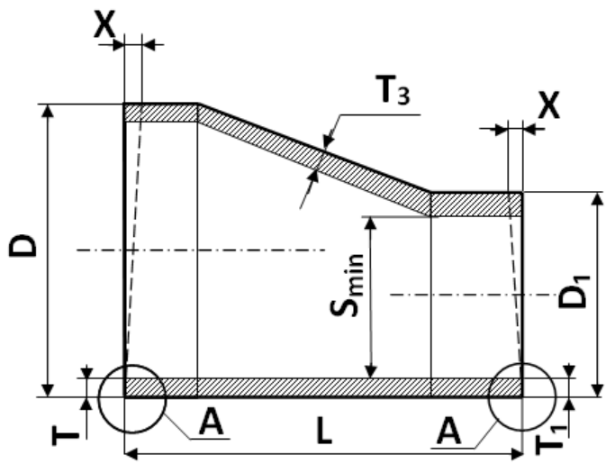
Redukcie excentrické / reducers excentric ASME B16.9
